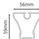
ПРОФИЛЬ ПОДДЕРЖКИ ТКАНИ Толщина: 2,5 мм
