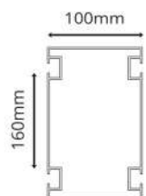
ПРОФИЛЬ КОЛОННЫ ТОЛЩИНА : 2mm
