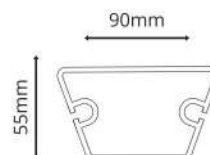
ПРОФИЛЬ СЪЕМНИКА Толщина: 2мм
