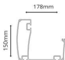
ПРОФИЛЬ ЖЕЛОБЫ Толщина: 3мм
