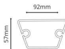
ПРОФИЛЬ СЪЕМНИКА Толщина: 3мм
