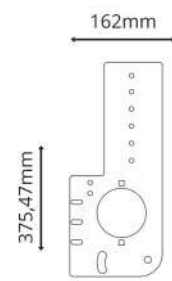
СТРОПИЛЬНЫЙ БОКОВОЙ ЛИСТ ТОЛЩИНА : 3mm
