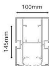
ПРОФИЛЬ СТРОПИЛЫ Толщина: 3мм
