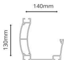
ПРОФИЛЬ ЖЕЛОБА Толщина: 2мм
