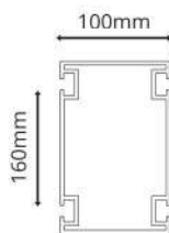
ПРОФИЛЬ КОЛОННЫ Толщина: 2мм
