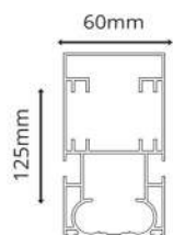
ПРОФИЛЬ СТПРОПИЛЫ Толщина: 2мм
