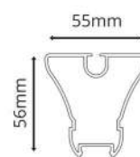
ПРОФИЛЬ ПОДДЕРЖКИ ТКАНИ ТОЛЩИНА 1.5
